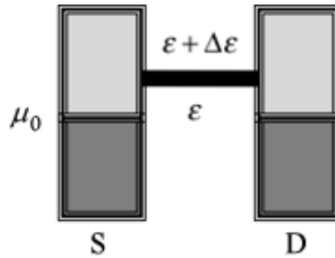
Рис. 8 – Модель дельта-термоэлектрика.
