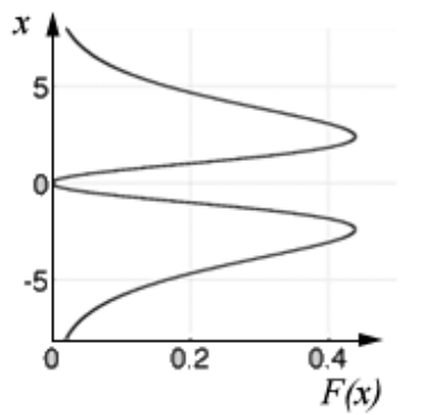
Рис. 10 – График функции F(x) = x^2 e^x / (e^x + 1)^2 .
