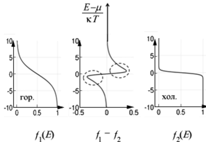
Рис. 2 – Два контакта, горячий и холодный, с одним и тем же значением \mu : разность фермиевских функций положительна для E > \mu и отрицательна для E < \mu .
